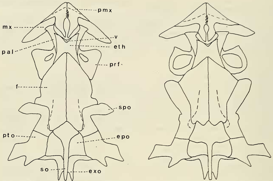
A. Marilynna pleurosticta (skull length 33 mm)
